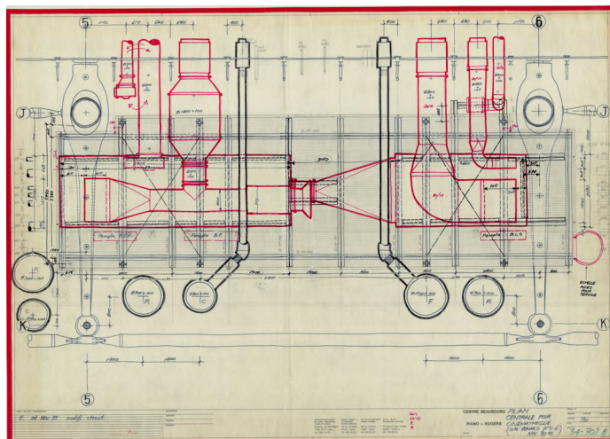
Piano+Rogers Architects (Shunji Ishida). Centre Beaubourg, aujourd'hui Centre Pompidou, projet définitif, plan de la centrale pour cinémathèque, s.d. [1974]. Rapidographe, feutre et crayon sur calque. Archives du Centre Pompidou, fonds des plans de la construction du plateau Beaubourg. Paris © Renzo Piano, Richard Rogers (avec l'aimable autorisation de Politecnico di Milano et Ruth Rogers)
